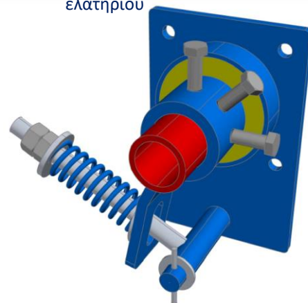
Βάση Στήριξης Mounting Base 225X150mm
